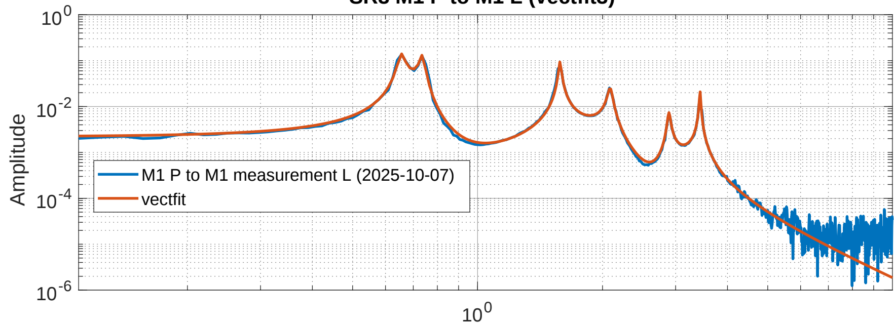
SR3 M1 P to M1 L (vectfit3)
