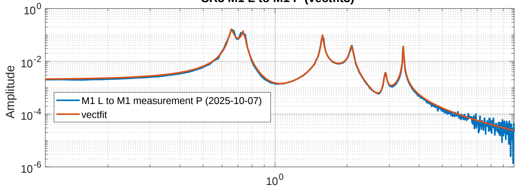
SR3 M1 L to M1 P (vectfit3)
