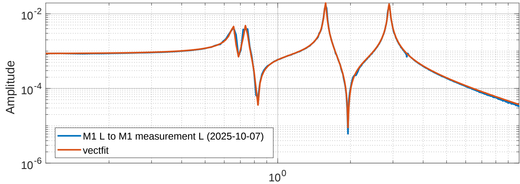
SR3 M1 L to M1 L (vectfit3)
